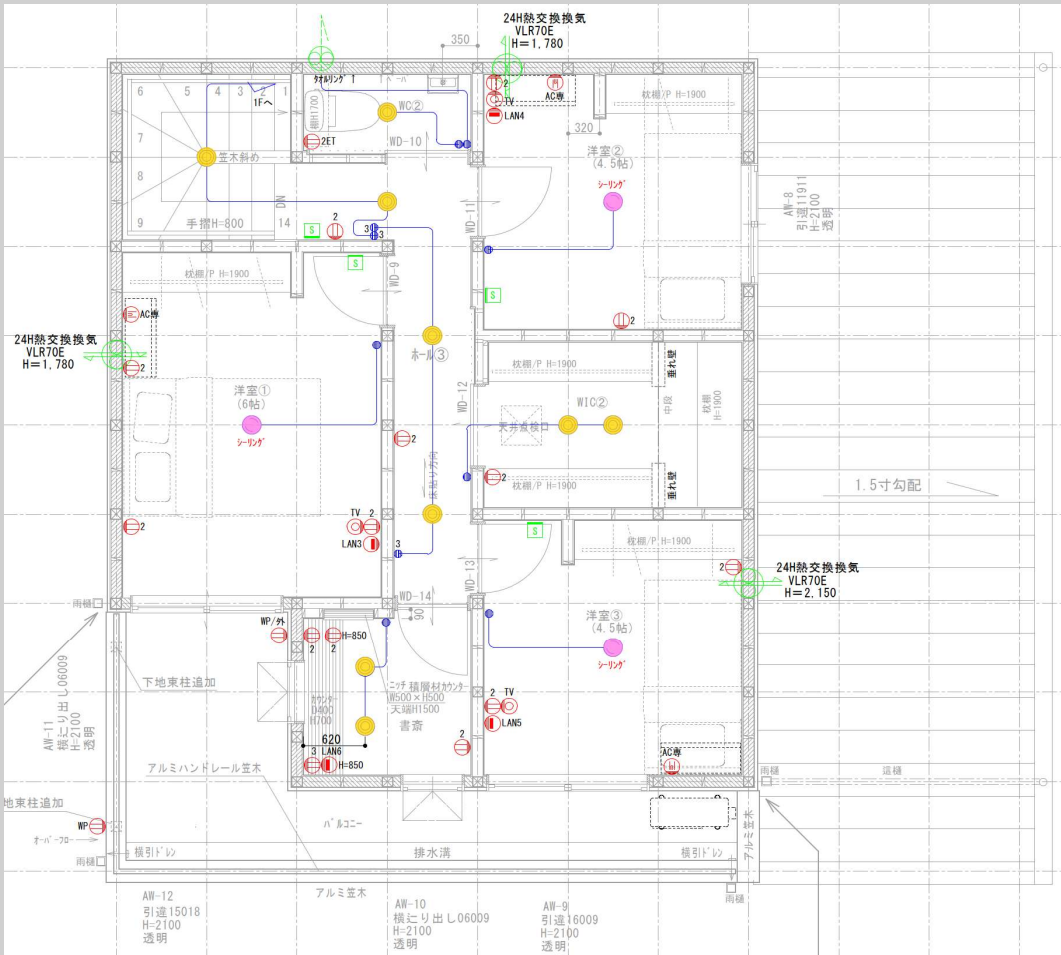
2階
