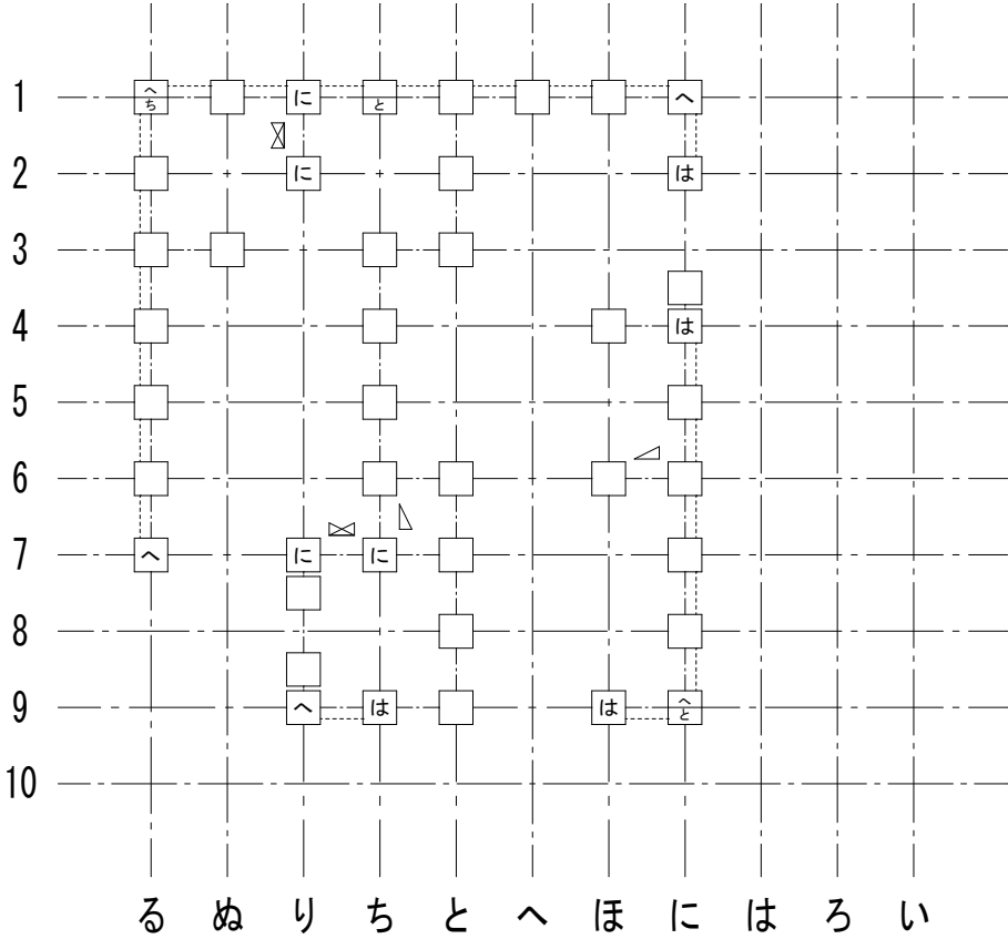
2階柱壁伏図
