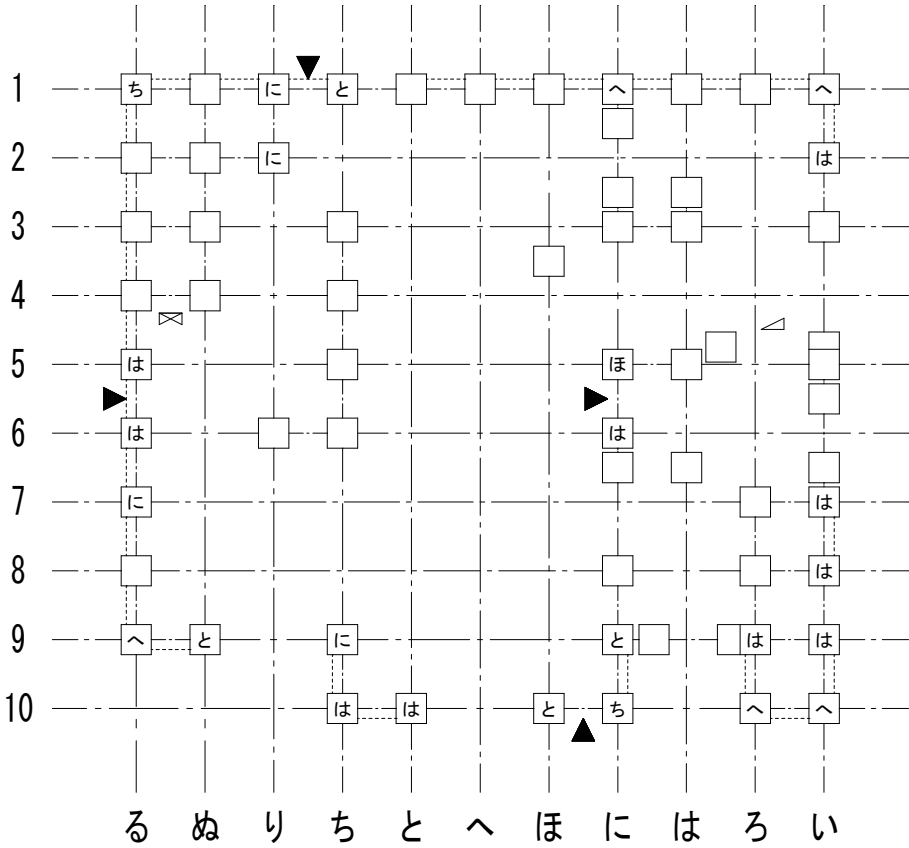
1階柱壁伏図
